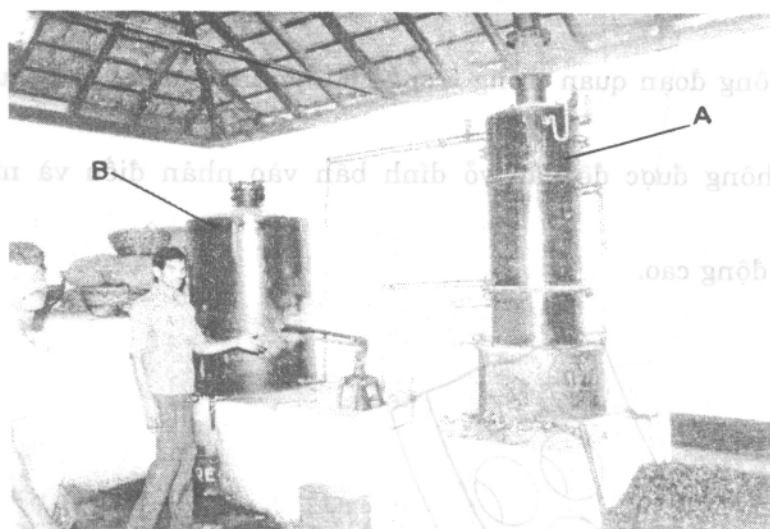
Hình 27: Nồi hấp sử dụng hơi nước 165 - 170^{\circ}\text{C} (Áp suất hơi 120 \text{ psi} \approx 8,76 \text{ kg/cm}^2 )
