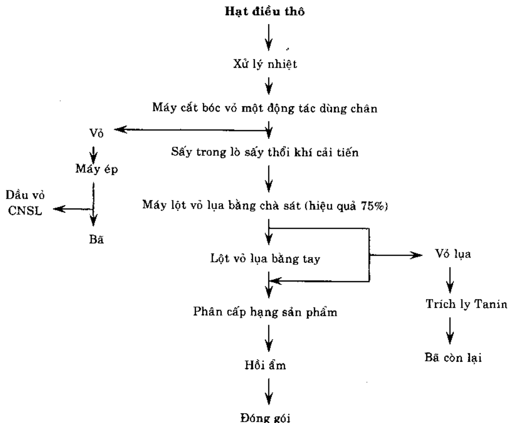
Sơ đồ 2 : Hệ thống chế biến hạt điều có mức độ cơ giới nhiều hơn.
