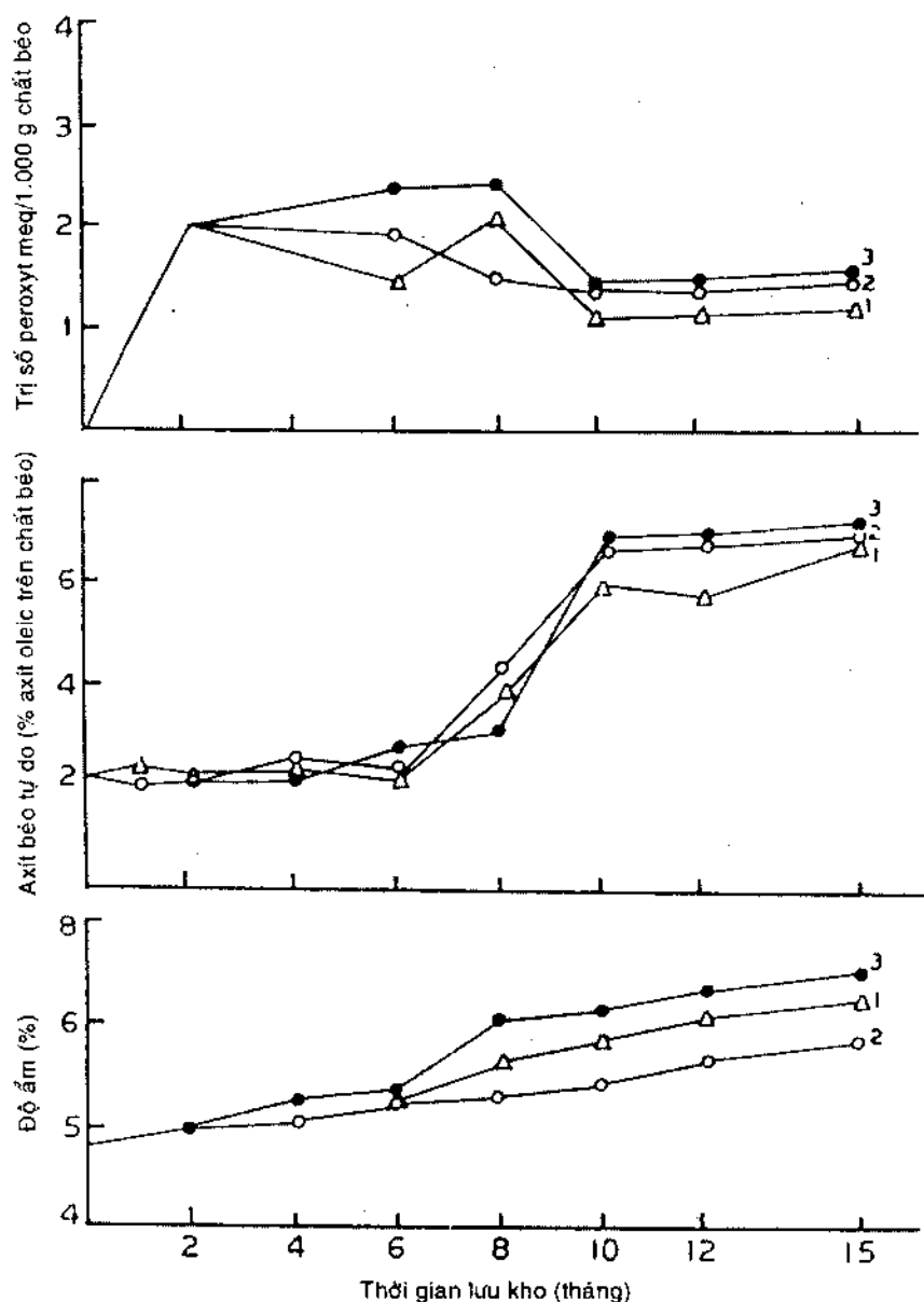
Hình 49: Những thay đổi độ ẩm, axit béo tự do và trị số peroxyt ở nhiệt độ phòng
