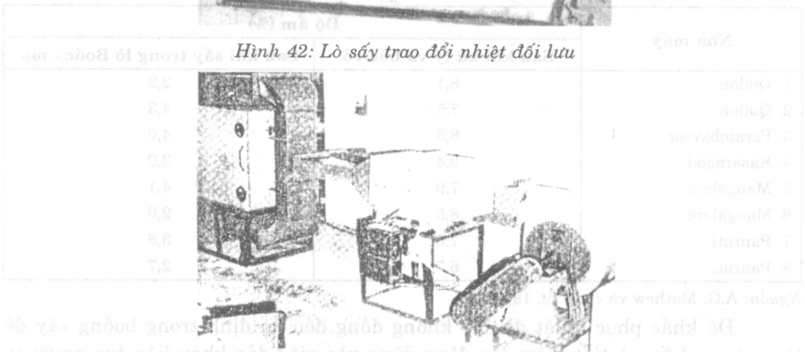
Hình 43: Lò sấy khí nóng tuần hoàn cưỡng bức kiểu thổi dọc (A.G. Mathew và cộng sự)
