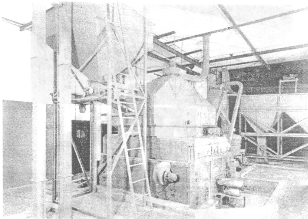
Hình 23 : Thiết bị chao dầu tự động kiểu băng tải của hãng Oltremare
