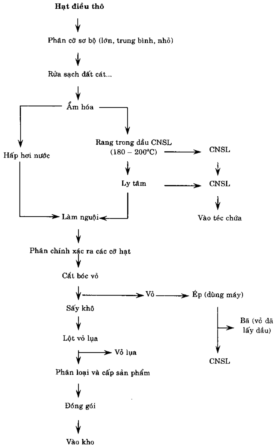
Sơ đồ 5 : Dây chuyền chế biến hạt điều
