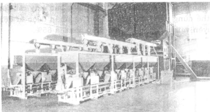
Hình 41: Hệ thống máy cắt tách bóc vỏ nạp liệu tự động kết hợp phân riêng nhân - vỏ (Oltremare)
