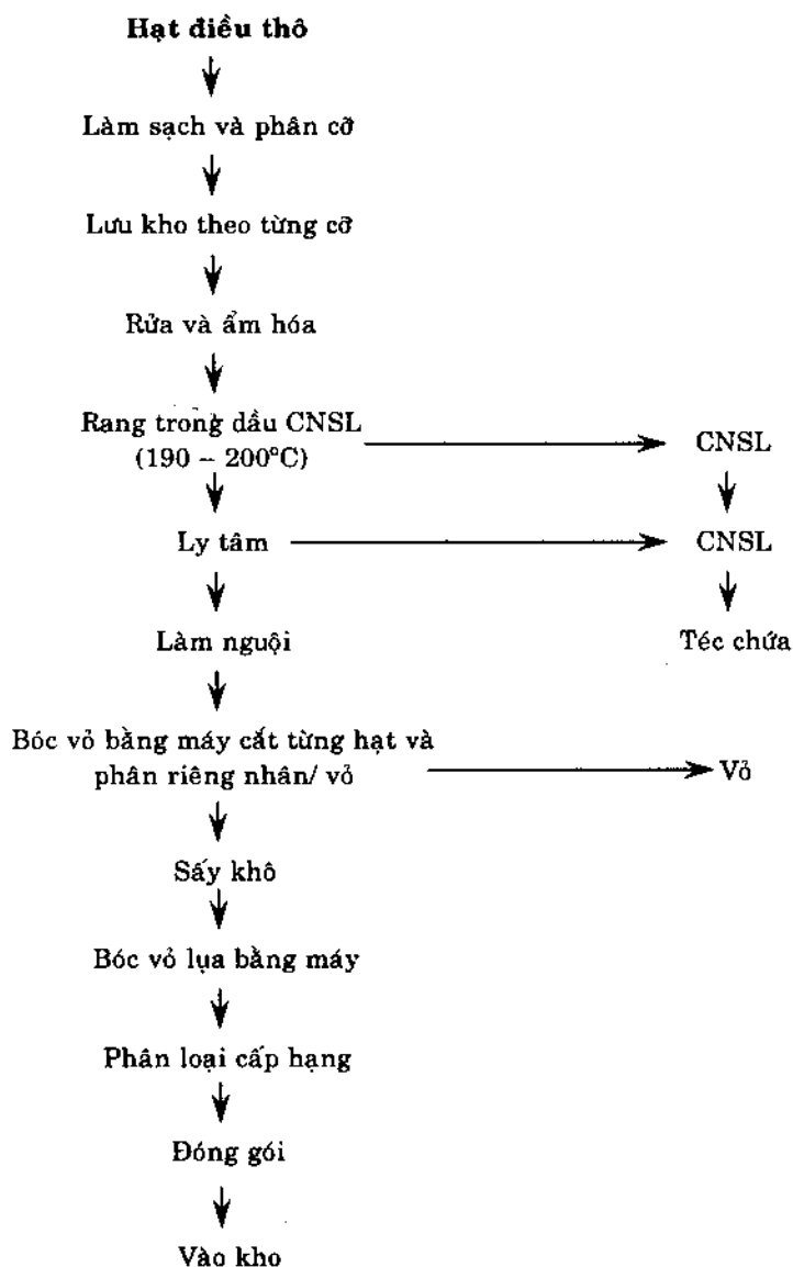
Sơ đồ 3: Hệ thống cơ giới Oltremare (Ý) (Single nut knife cutting)
