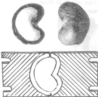
Hình 33: Hai lưỡi dao mài theo kích cỡ hạt điều
