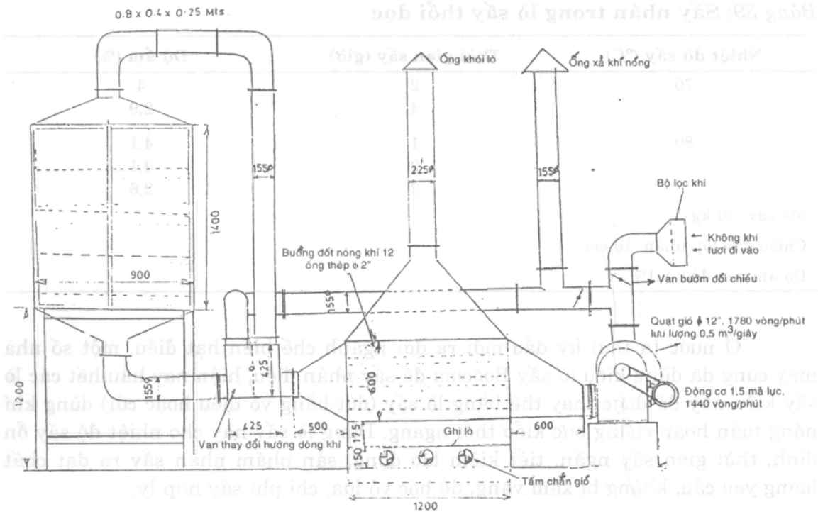
Hình 44: Sơ đồ lò sấy khí nóng tuần hoàn cưỡng bức kiểu thổi dọc (A.G.Mathew và cộng sự.)
