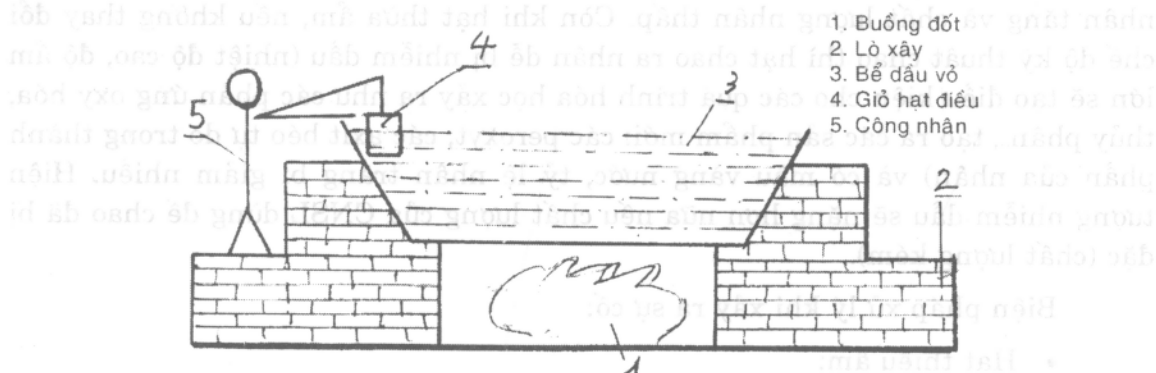
Hình 22: Lò chao dầu thủ công
