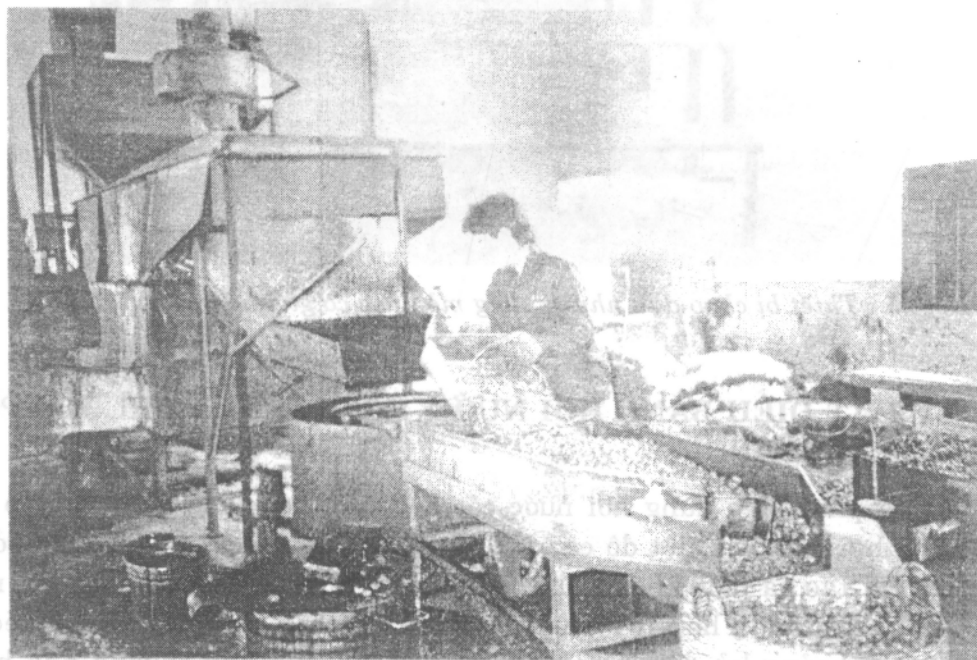
Hình 24 : Thiết bị chao dầu cơ giới bán tự động kiểu băng tải của Việt Nam
