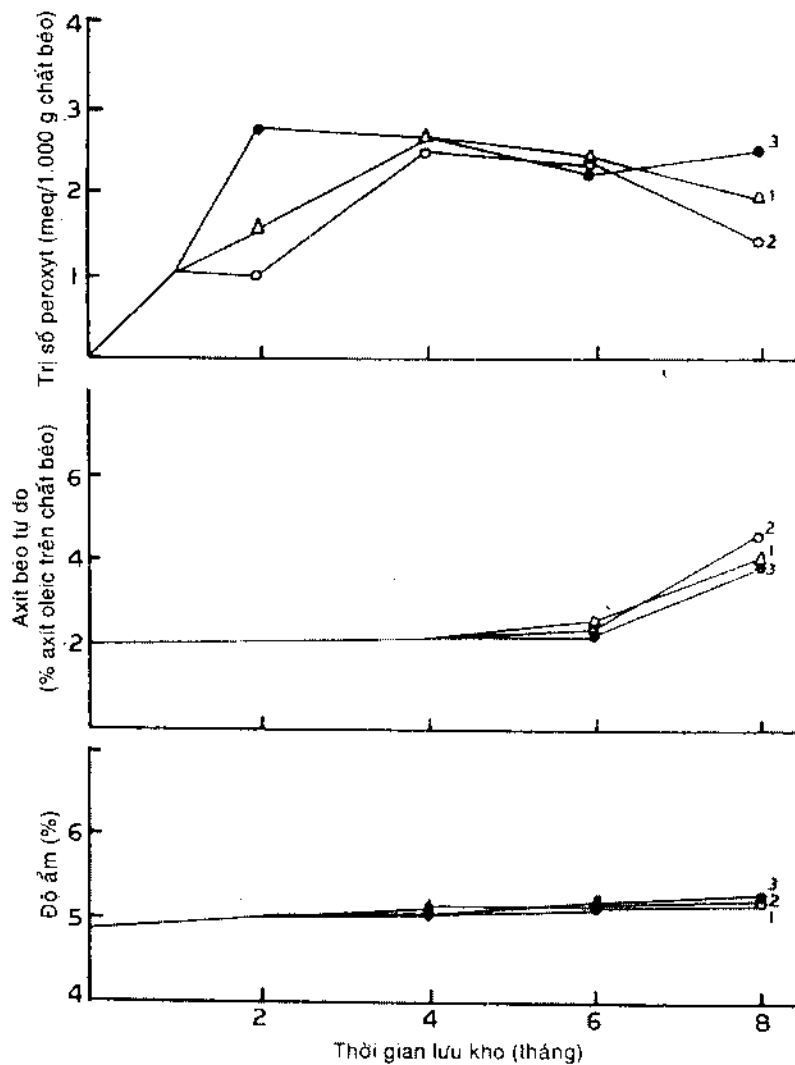
Hình 50: Những thay đổi độ ẩm, axit béo tự do và trị số peroxyt ở nhiệt độ 37°C.
