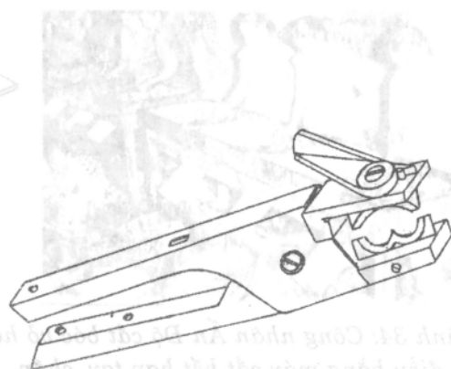
Hình 38b: Kẹp bóc vỏ hạt điều (Pháp)
