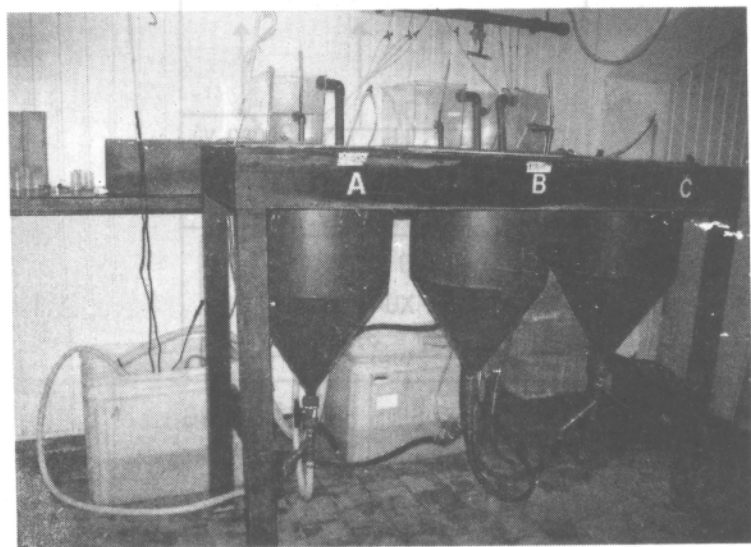
Hình 5. Hệ thống nuôi ấu trùng Tôm Càng Xanh M.rosenbergii theo qui trình tuần hoàn kín
