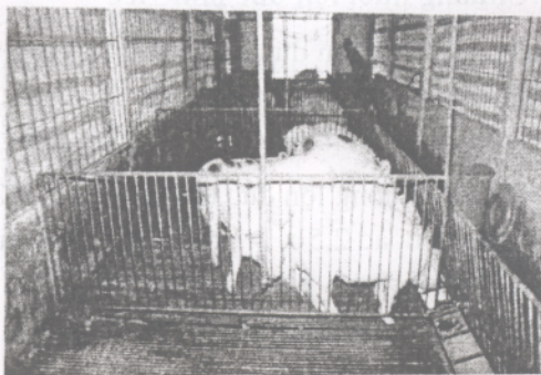
Chuồng lợn choai với sàn bằng thép \Phi 8, máng ăn bằng nhựa PVC có chia ngăn.
