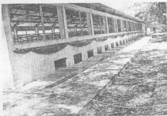
Chuồng lợn nái đẻ và nuôi con có hệ thống bạt che
