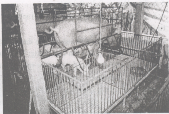
Cũi lợn nái đẻ và nuôi con trong nông hộ tại Hà tây (lợn mẹ trên sàn bê tông, lợn con trên sàn nhựa)
