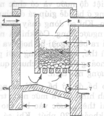
Hình 2.8: Hệ thống lọc cơ học theo Woynarowich, (1975).
