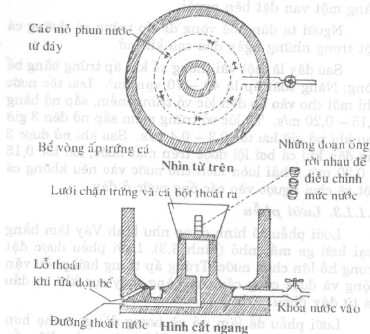
Hình 3.2: Bể vòng để ấp trứng cá, nhìn từ trên xuống và hình cắt ngang từ một bên
