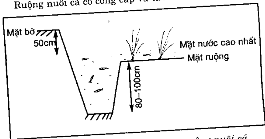
Hình 17. Sơ đồ thiết kế xây dựng ruộng nuôi cá
