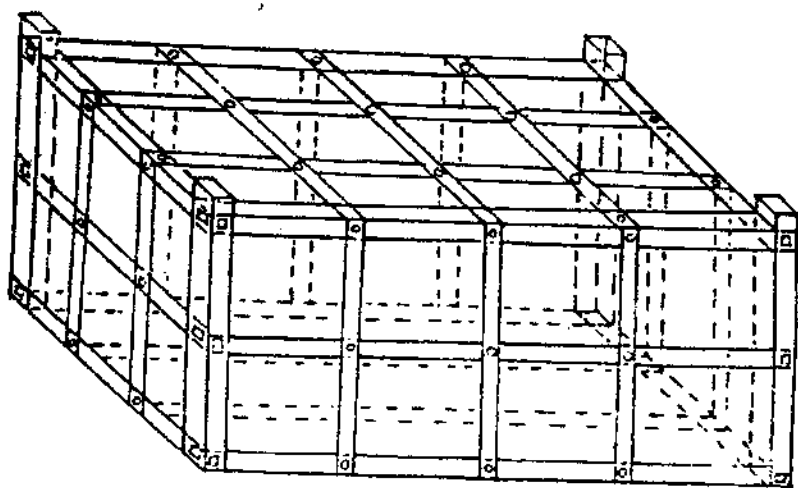
Hình 19. Kết cấu khung lồng bằng gỗ
