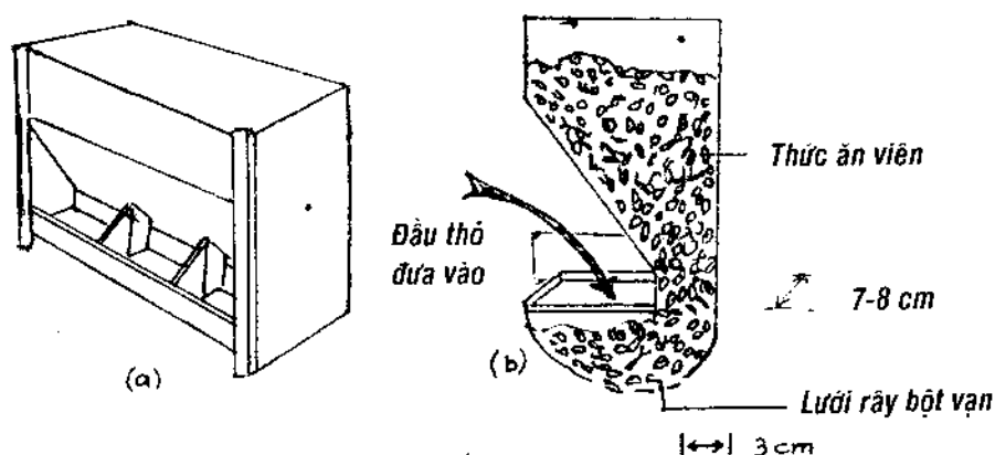
Hình 2 : Máng ăn thức ăn viên : (a) phôi cảnh (b) mặt cắt bên
