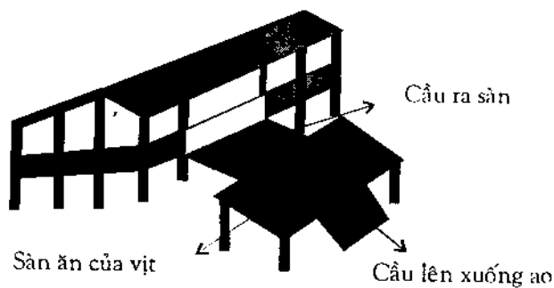
CHUỒNG NUÔI VỊT ĐẼ (Chuồng trên bờ ao, sàn trên mặt ao)
