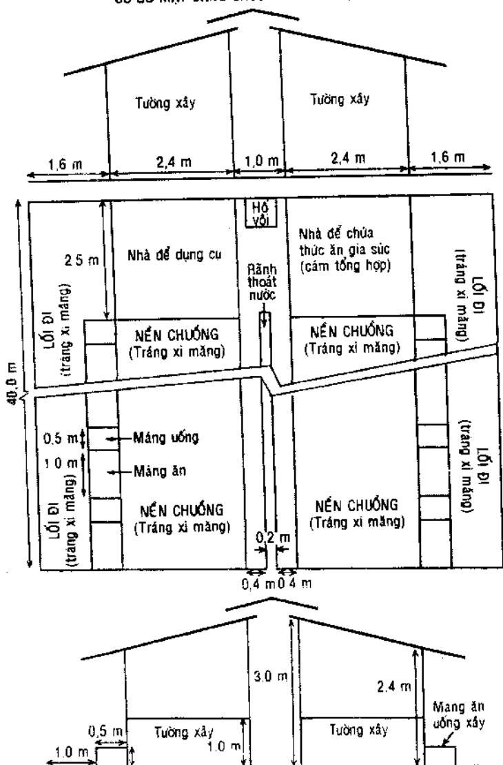
SƠ ĐỒ MẶT BẰNG CHUỒNG NUÔI BÒ (50 CON)
