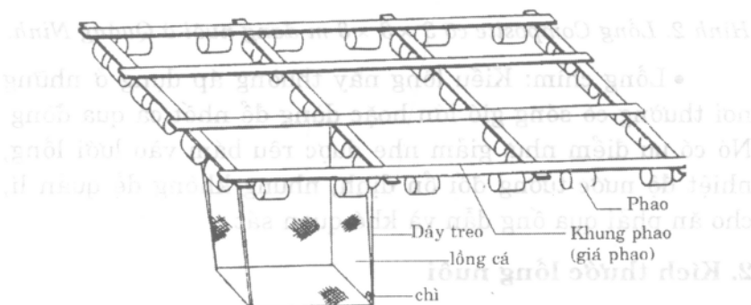
Hình 3. Sơ đồ mô hình lồng nổi (1 bè cá có 9 lồng cỡ 3 \times 3 \times 3 m).
