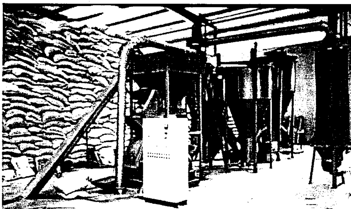
Dây chuyền chế biến thức ăn gia súc quy mô 3 tấn/giờ
