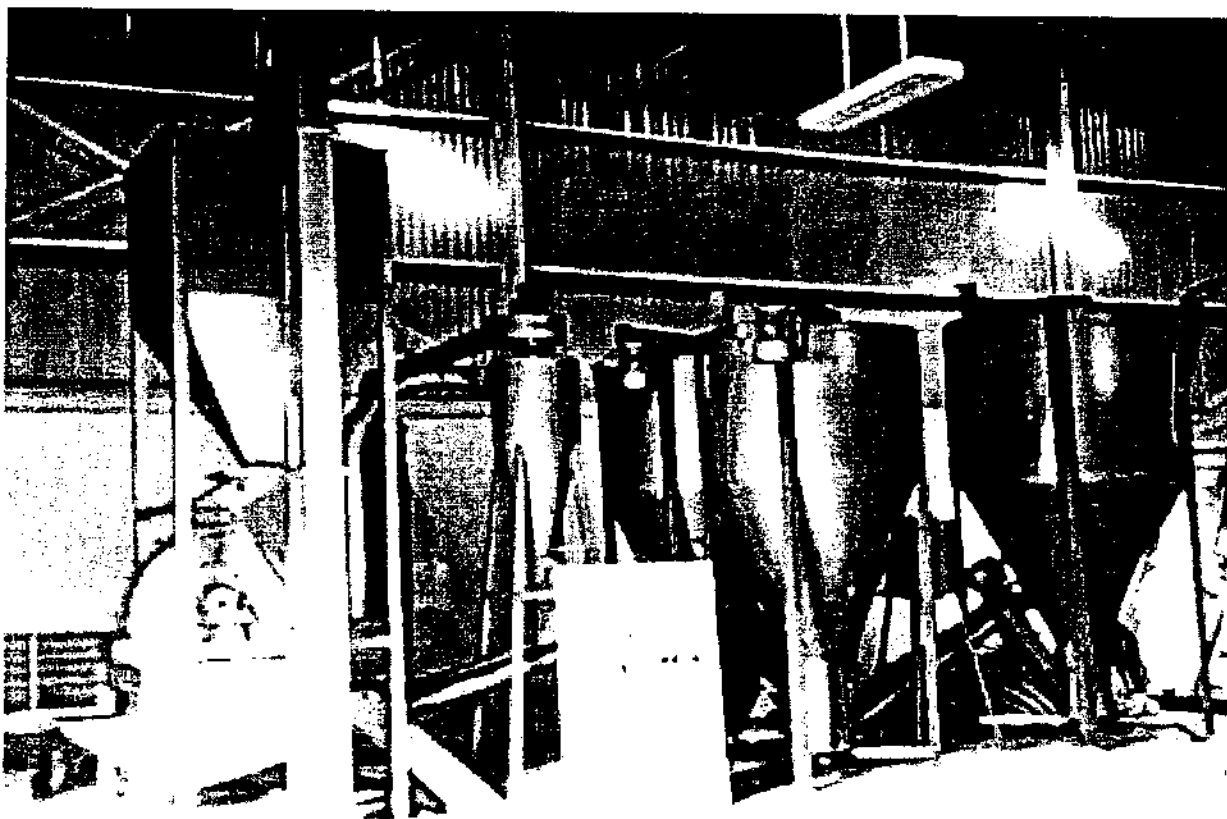
Dây chuyền chế biến thức ăn gia súc quy mô 5 tấn/giờ
