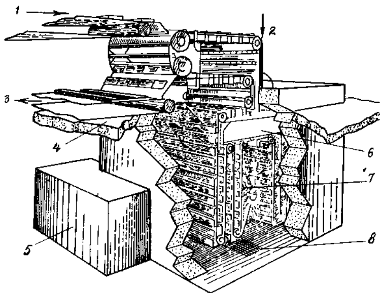
Hình 9. Sơ đồ hệ thống chiếu xạ thực phẩm
