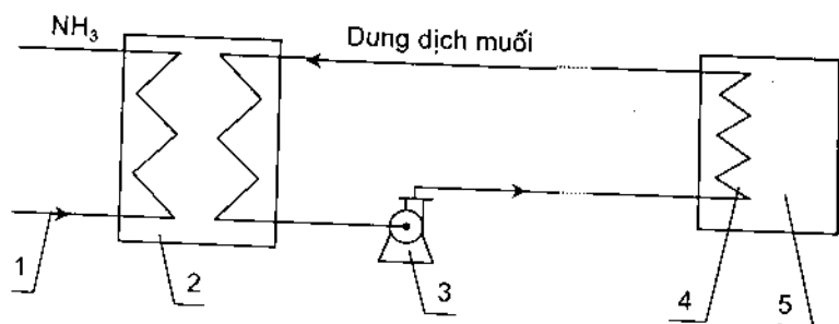
Hình 4. Sơ đồ hệ thống làm lạnh gián tiếp qua chất tải lạnh
