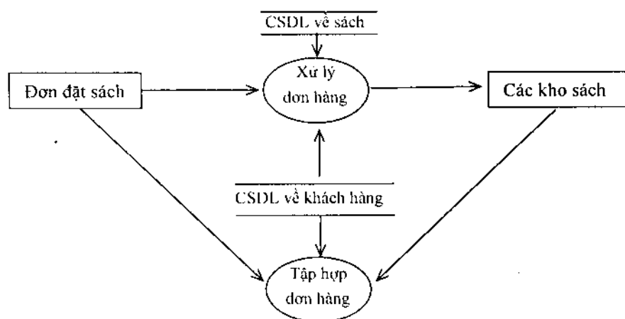
Hình 1-4. Sơ đồ dòng dữ liệu trong hệ xử lý đơn đặt hàng
