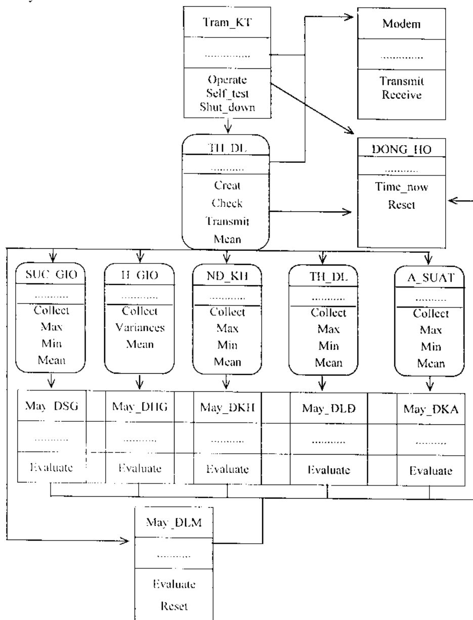
Hình 2-8. Cấu trúc hệ thống khí tượng thủy văn
