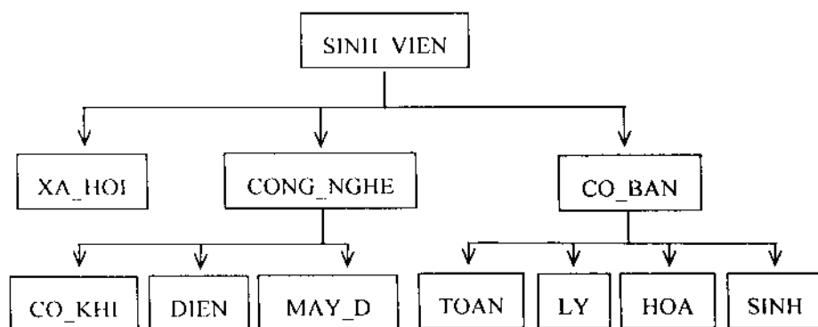
Hình 3.4. Cấu trúc phân cấp các lớp trong quân hệ kế thừa
