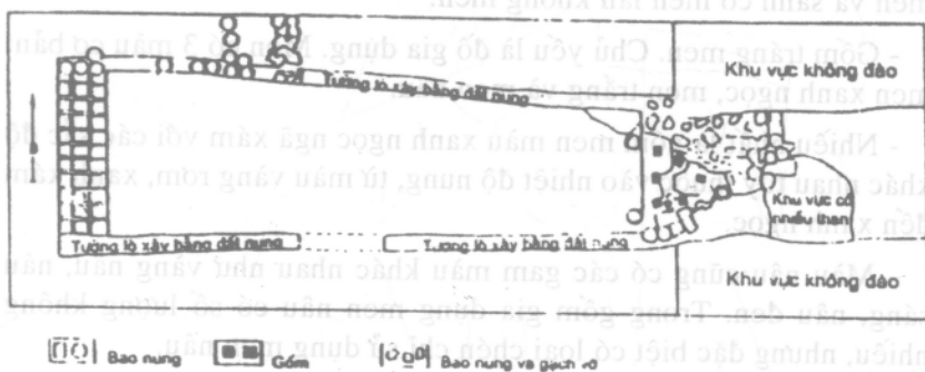
Bản vẽ 47: Bình đồ lò gốm Gò Cây Me
