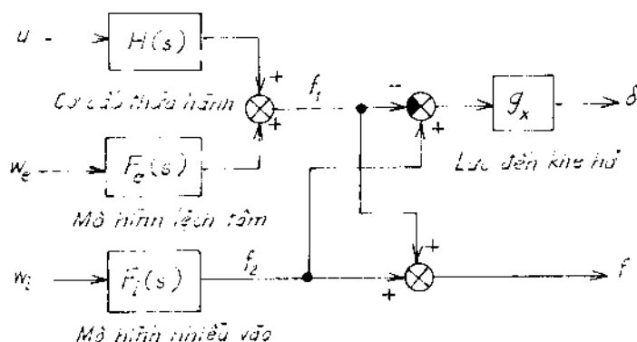
Hình 9.12. u - điều khiển ; \delta - độ dày ; f - lực tăng ở trục cán; w_1 , w_2 - ổn trắng đối với mô hình của nhiễu.
