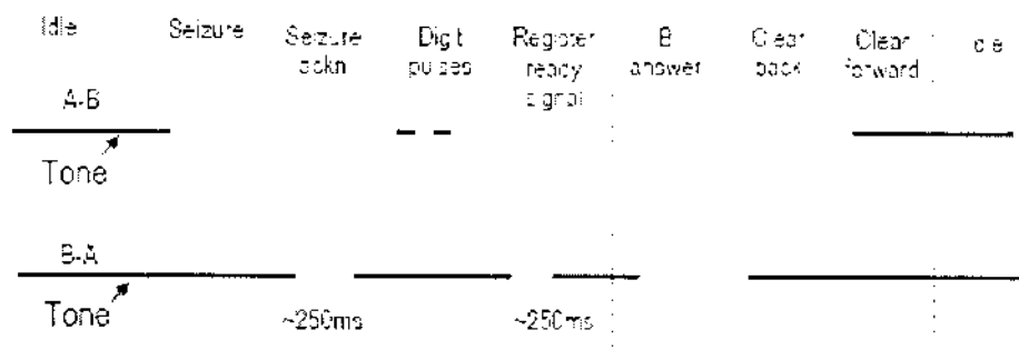
Hình 4-10: Ví dụ về hệ thống tín hiệu AC.
