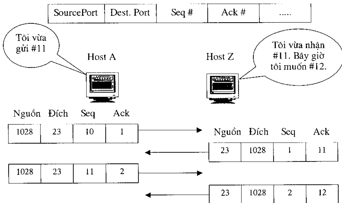
Hình 7-25: Số Acknowledgment.
