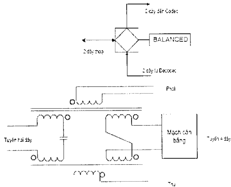
Hình 5-6: Hybrid.
