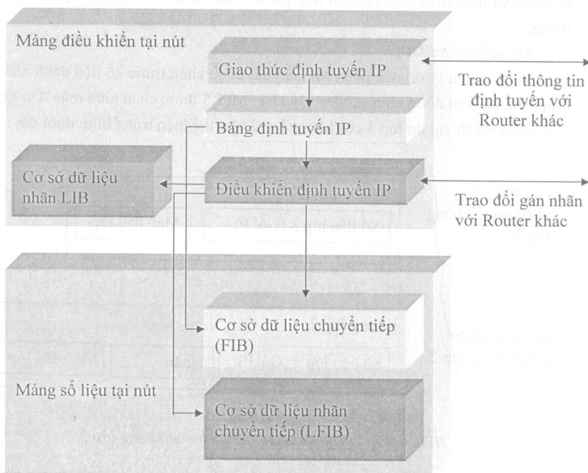
Hình 8-16: Cấu trúc LSR biên trong chế độ hoạt động khung.
