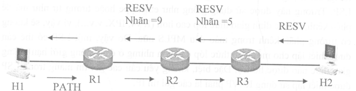
Hình 8-24: Nhãn phân phối trong bảng tin RSVP.
