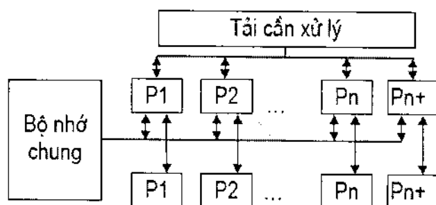
Hình 3-14: Dự phòng n+1 .
