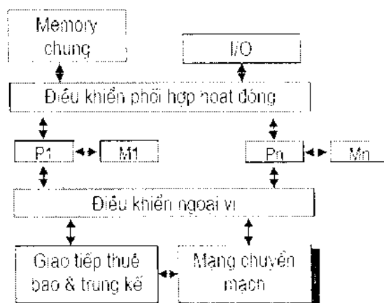
Hình 3-3: Điều khiển tập trung.
