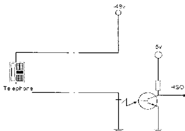
Hình 5-4: Supervision.
