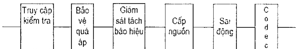
Hình 5-10: Giao tiếp trung kế tương tự.
