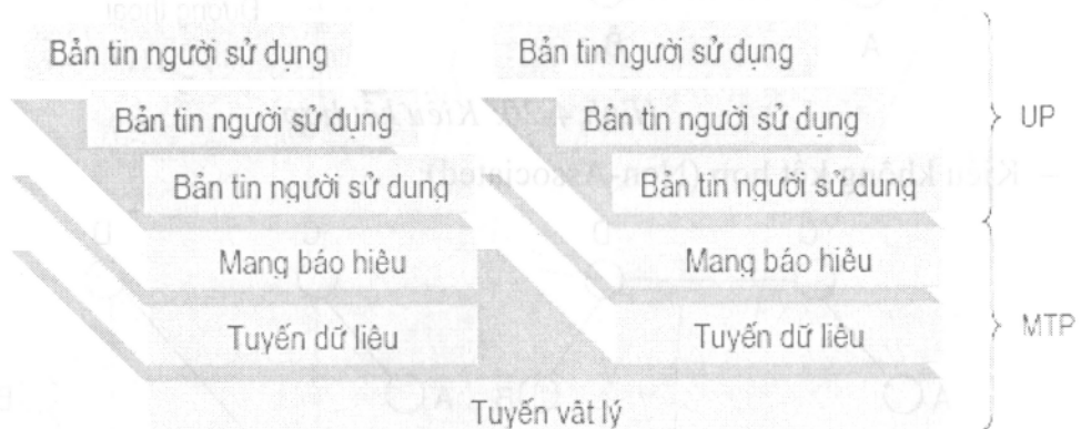
Hình 4-23: Cấu trúc 4 mức của báo hiệu số 7.
