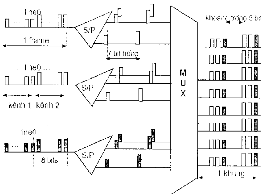
Hình 2-13: Ghép 3 tuyến PCM S/P.
