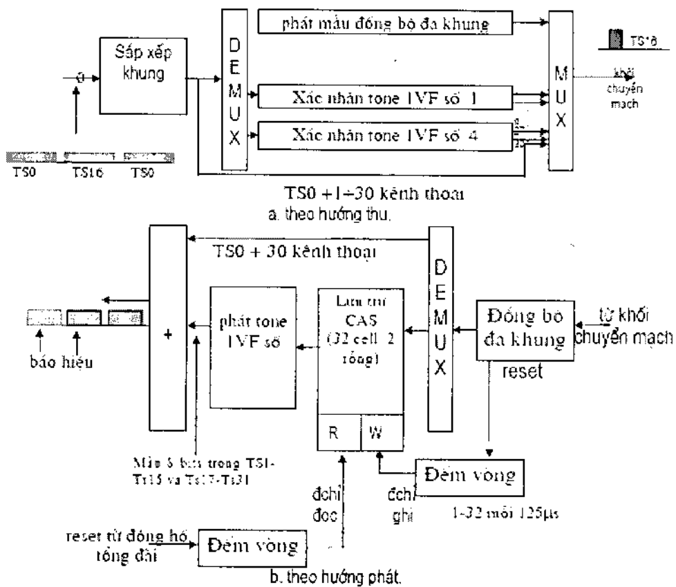
Hình 4-38: Chuyển đổi IVF sang CAS.
