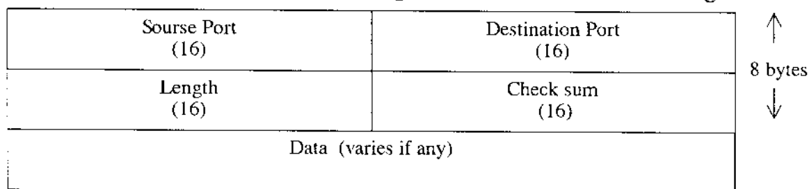
Hình 7-22: UDP header.
