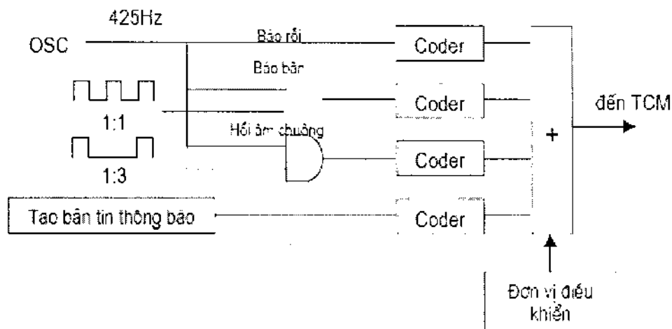
Hình 4-40: Sử dụng kỹ thuật tương tự.
