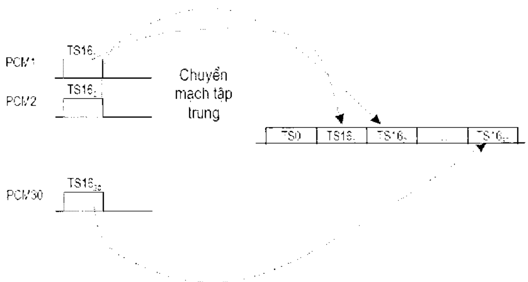
Hình 4-34: Ghép kênh tín hiệu báo hiệu tại chuyển mạch tập trung.
