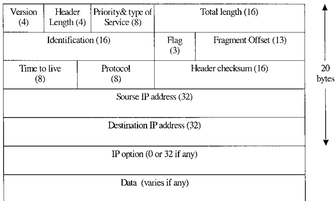
Hình 7-27: Minh họa các trường thông tin của IP header.
