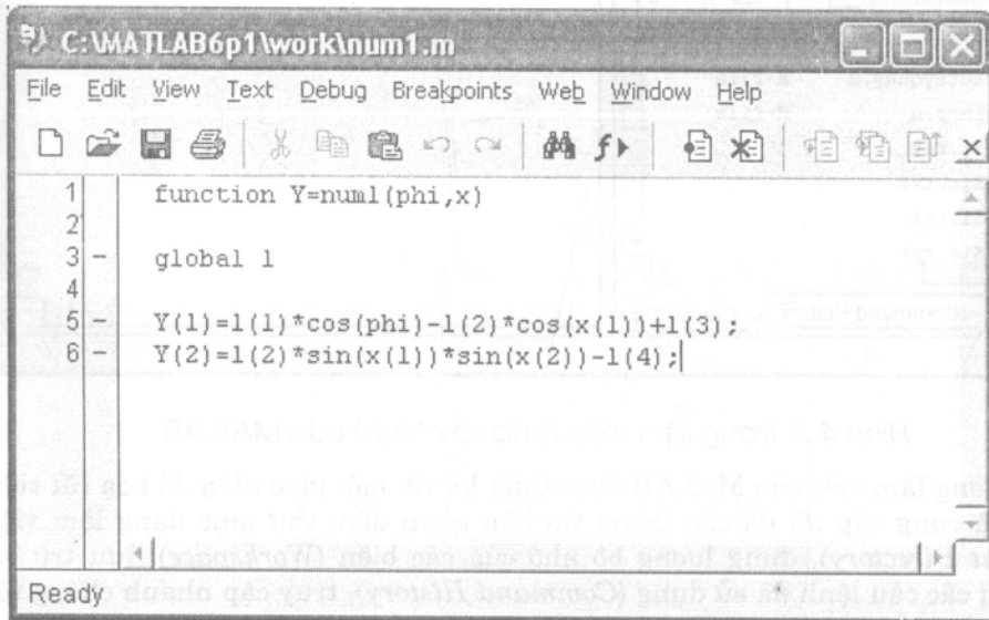
Hình 4.8: MATLAB -Editor
