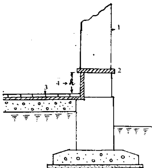
H.4. Lớp cách ly cơ học
